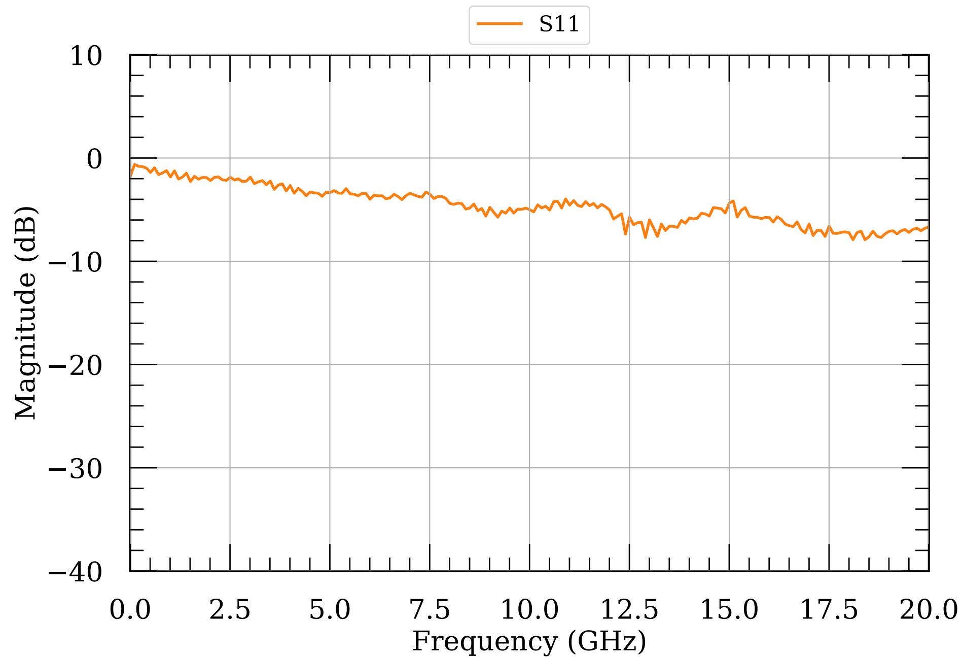
LNA S-params module034
